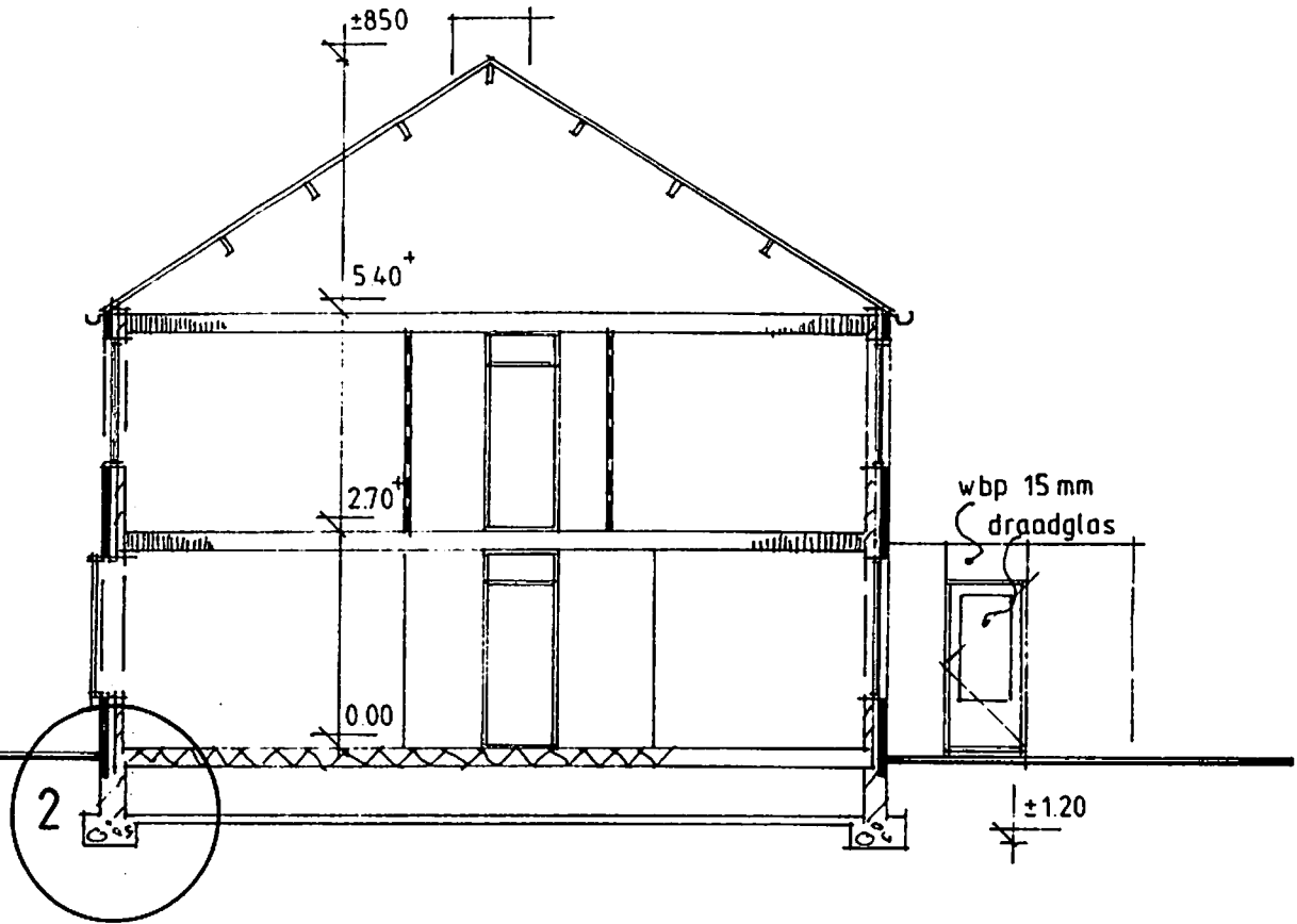
doorsnede A
